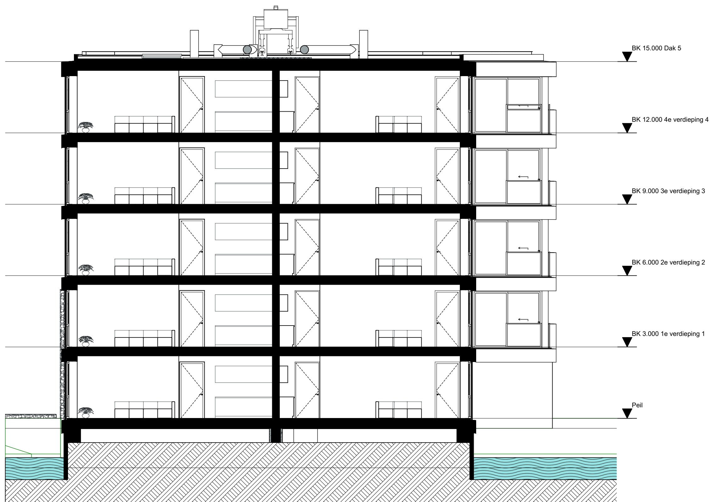
Doorsnede B-B
