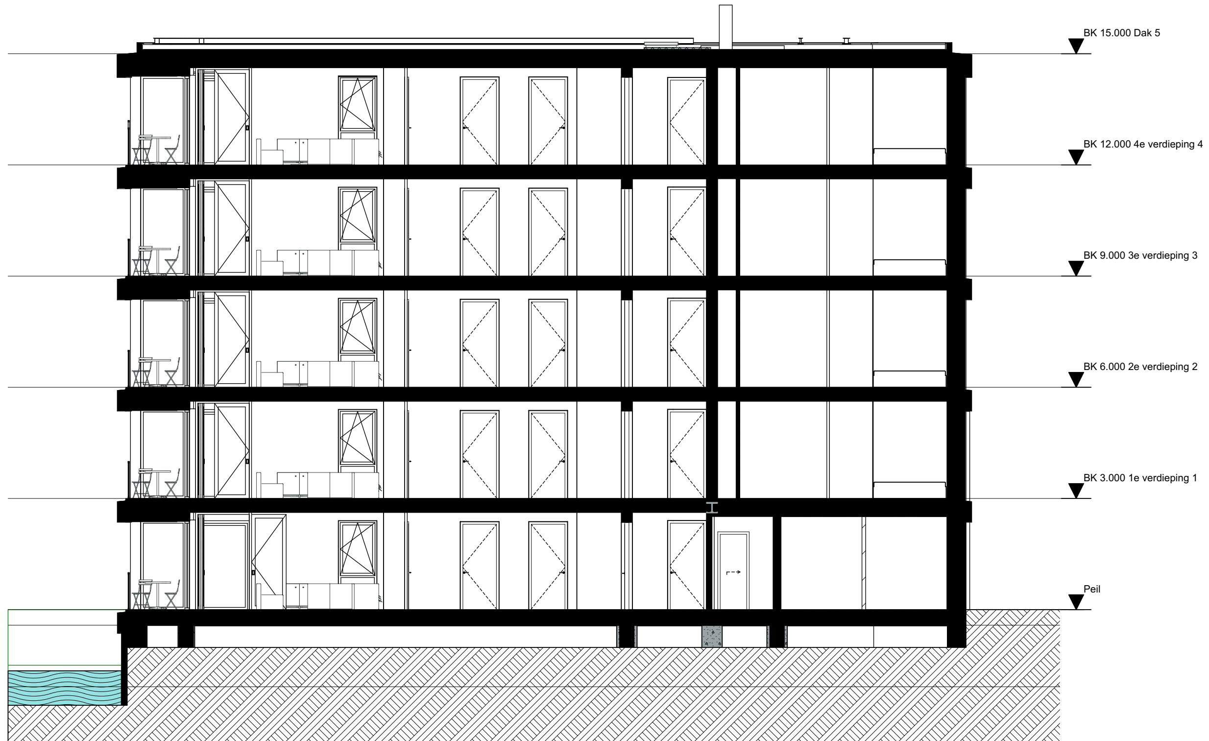
Doorsnede A-A
